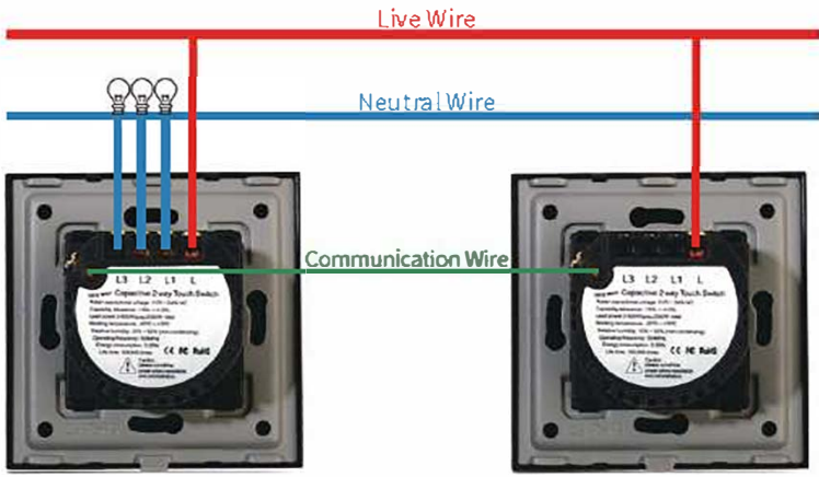
2way wiring
