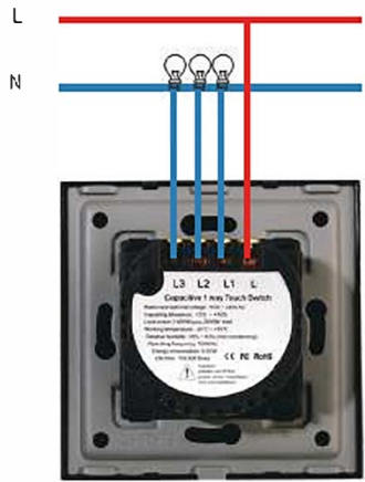
1way/Bell wiring
